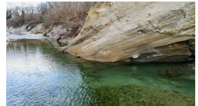
Stratificazioni in evidenza lungo lo Stirone
